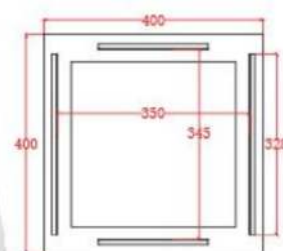
ramka osłonowa lampy CANOPY
